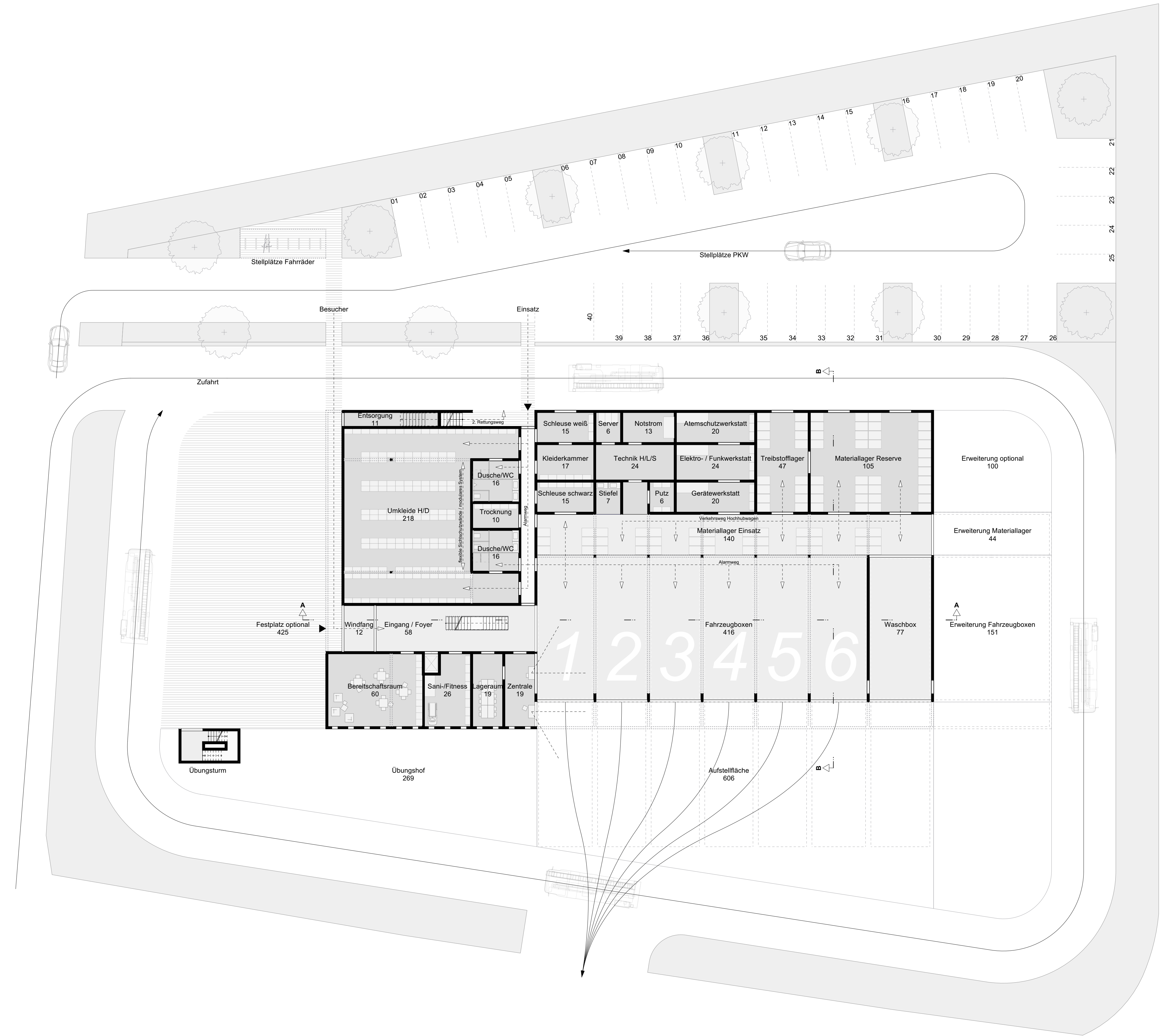
Grundriss EG | 1:200
